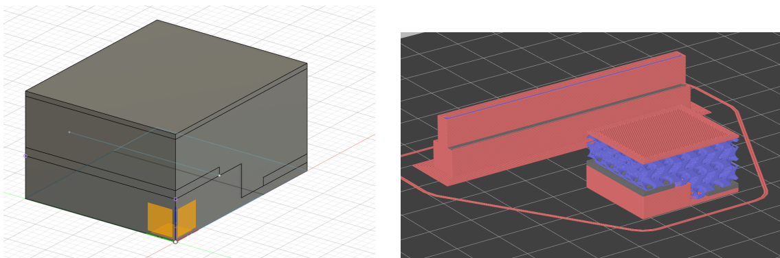
Figure 4. Différentes étapes de la pièce. la perspective cavalière en CAO (gauche). vue dans le slicer après découpage (droite). La pièce allongée visible à côté du capteur est la tour de nettoyage, utilisée pour purger les résidus de filament lors des changements de matériau.
